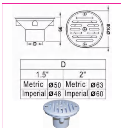
BW1424 池壁回水器 Wall return
