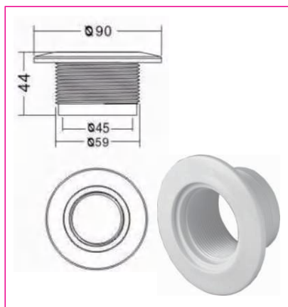
BW2022 真空吸污配件 Suction fitting
