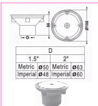
BW1425 池壁回水器 Wall return
