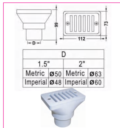
BW1019 渠盖排水器 Gutter drain
